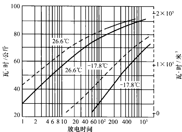
图 13.1 银-锌电池的性能
