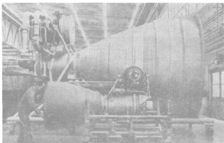
图 3.7 F-1 型发动机的外形 (里面的是 F-1 的原尺寸模型,外面的是 H-1 发动机)
