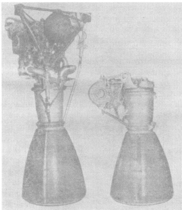
图 3.4 86 吨推力发动机的外形
