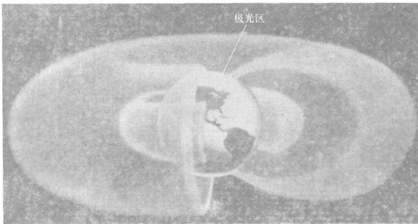
图 1.7 地球的内外辐射带
