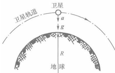
图 12.1 卫星的失重
