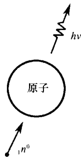
图 11.7 中子的 \gamma 吸收
