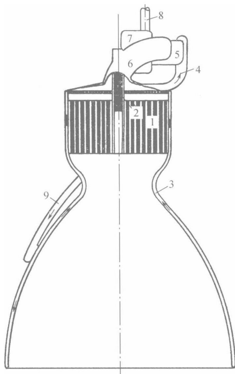
图 7.1 原子火箭发动机
