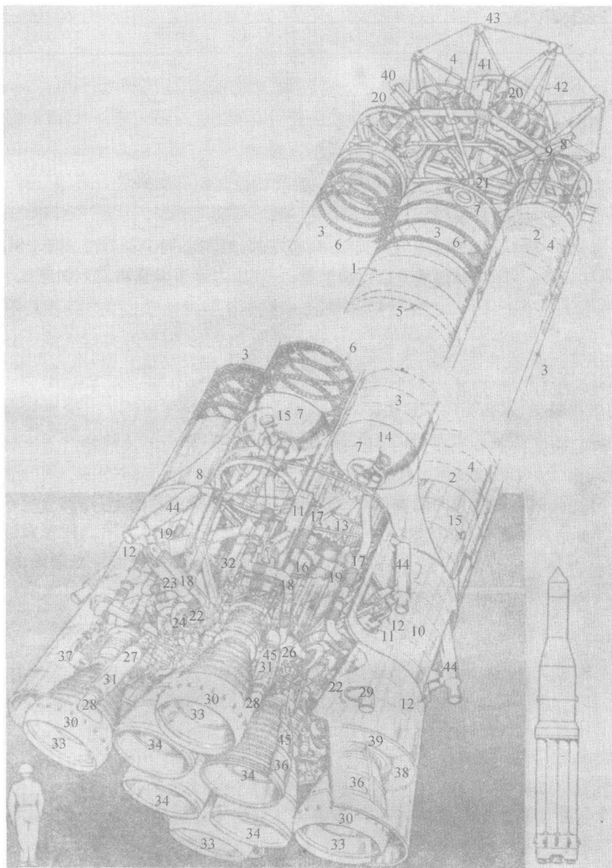
图 4.5 “土星”火箭第一级的结构详图
