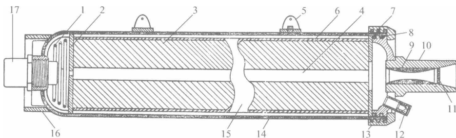
图 2.2 典型的固体推进剂起动火箭发动机的剖面图
