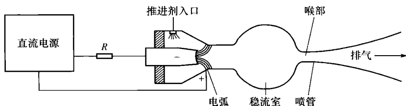
图 7.3 电弧火箭发动机
