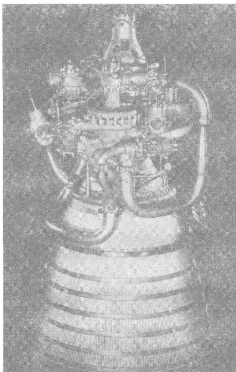
图 3.9 LR-115 型发动机的外形
