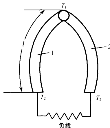
图 13.11 热电偶电路
