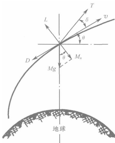
图 5.2 起飞轨道上火箭受力图
