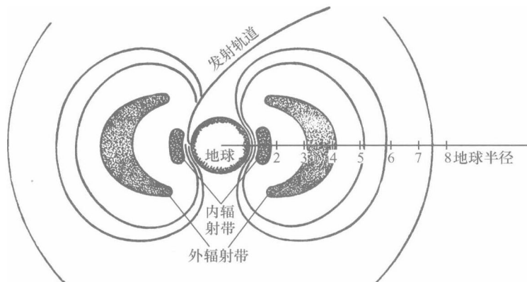
图 11.9 绕过内外辐射带的航行轨道
