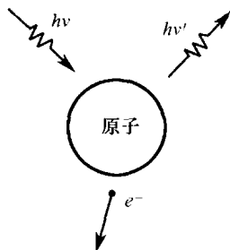
图 11.2 康普顿散射
